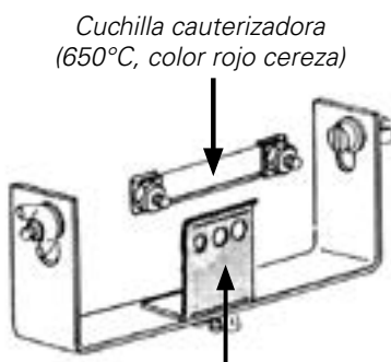
Placa guía con orificios
